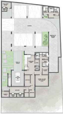
BASEMENT 9,538 SQ.FT
